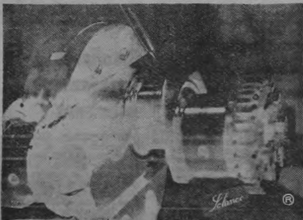
ESTA PIEZA, de la que la fotografía apenas capta una parte, es el eje principal de impulsión a la hélice. El eje vale 7500 colones. La ALPA ha perdido varios de ellos arruinados por la arena volcánica.
